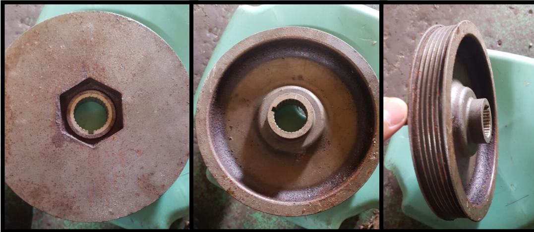
A3 (175 ~ 225 HP) 13811-ZY3-000 (PULLEY, CRANKSHAFT)
