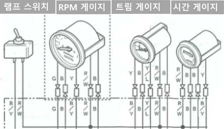
게이지 배선도
