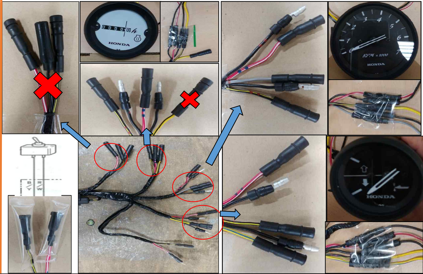
게이지 배선 연결 사진
